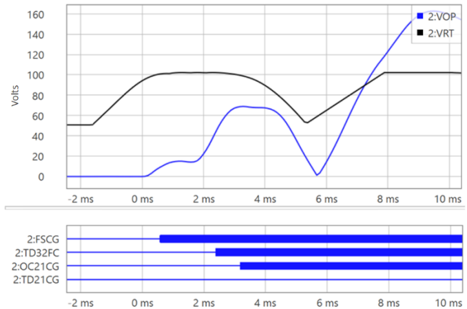
Fig. 26. Sam TD21CG restrains.
